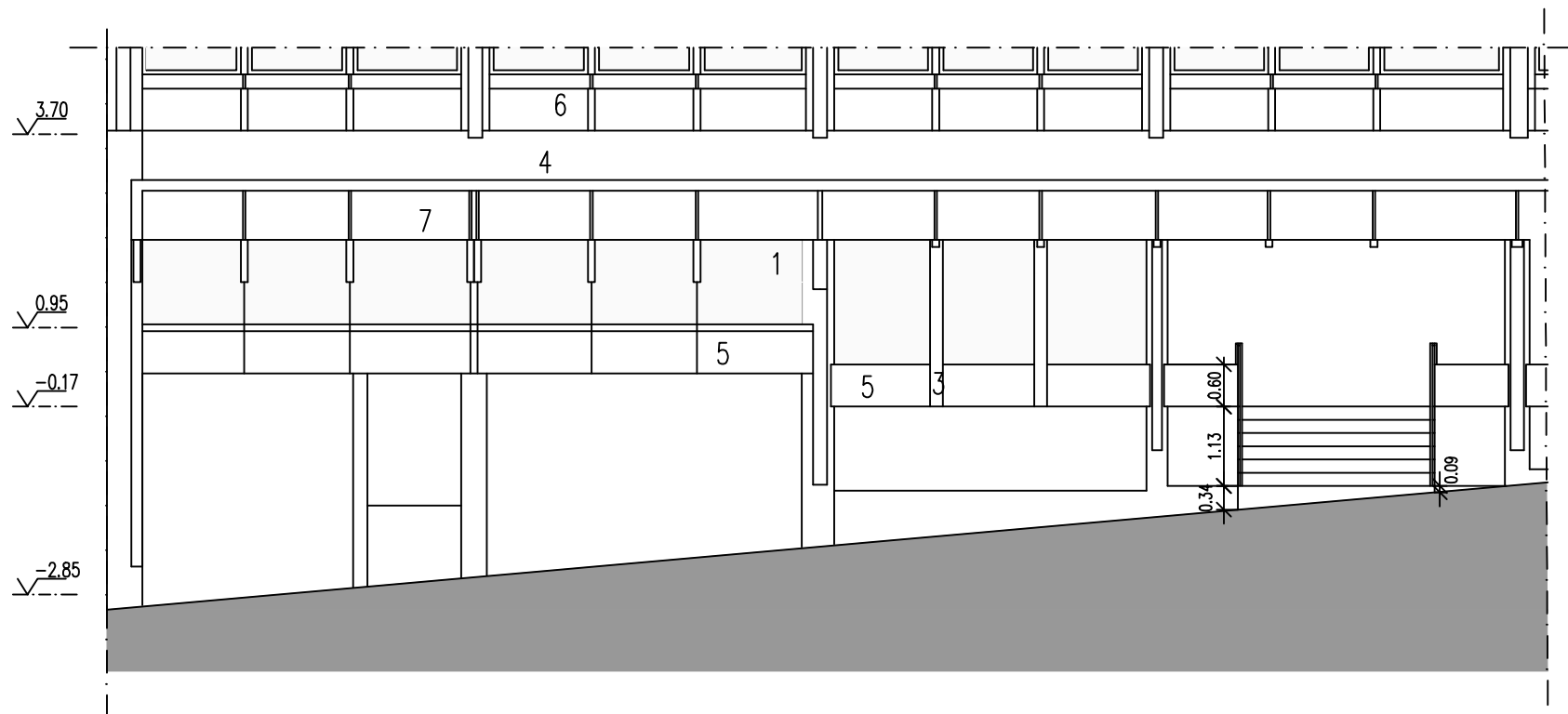
ALÇADO PRINCIPAL
