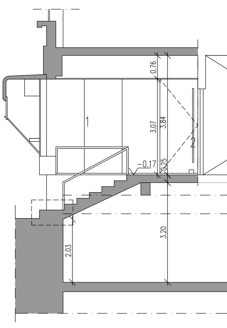
CORTE AB
