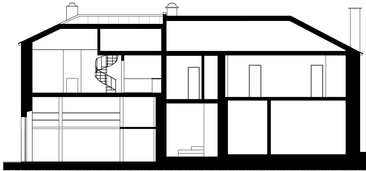
CORTE AB
